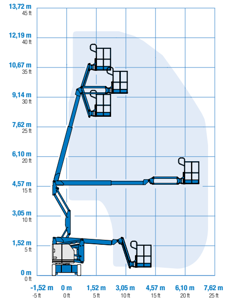
Arbeitsdiagramm Z-34/22N
